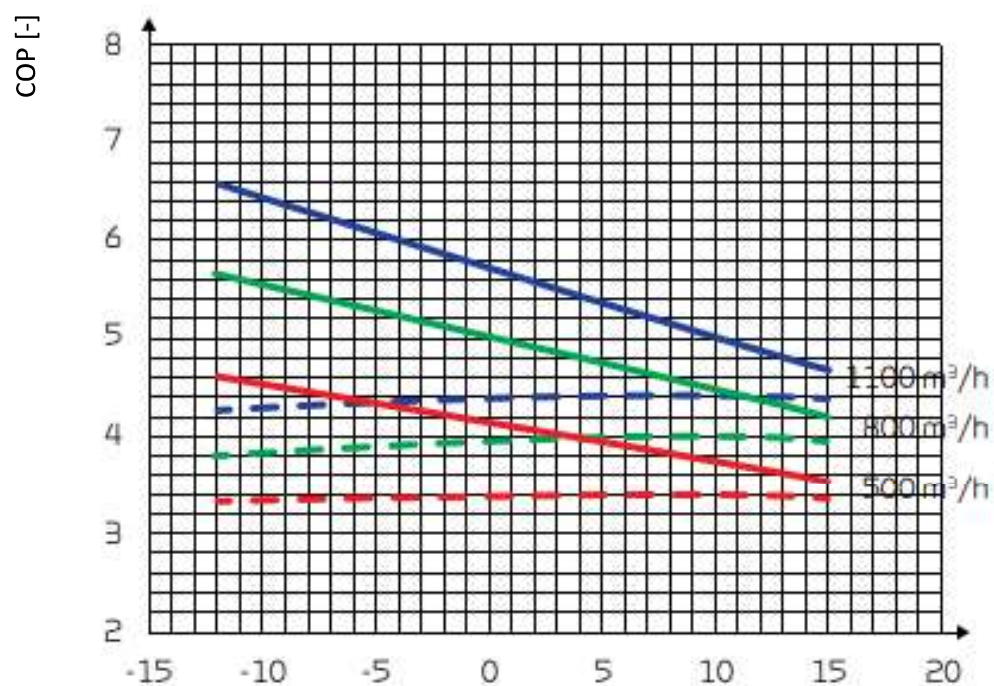
COP (EN14511), odťah 21 °C
